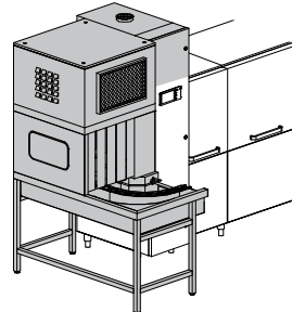
HDRA 218M Asciugatura Elettrica 4.5 Kw su curva motorizzata 180° + Recuperatore Termico Electric Dryer 4.5 Kw on 180° motorized arc + Heat Recovery
