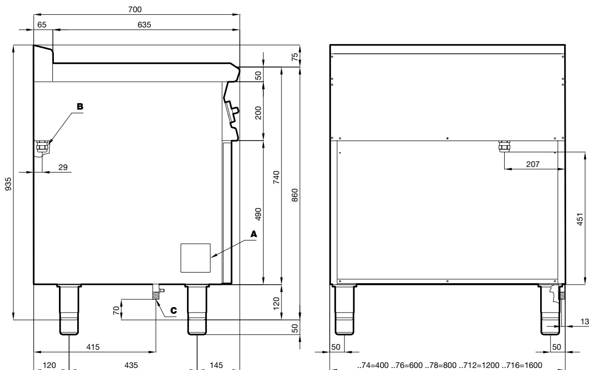
A Targhetta caratteristica / Data plate / Typenschild Plaque des caractéristiques / Chapa de características
